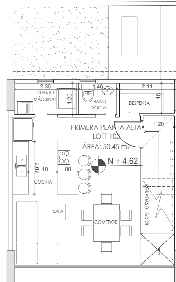
PRIMERA PLANTA ALTA
