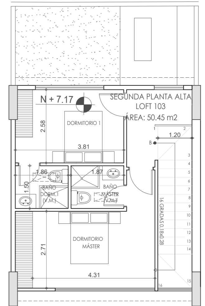
SEGUNDA PLANTA ALTA
