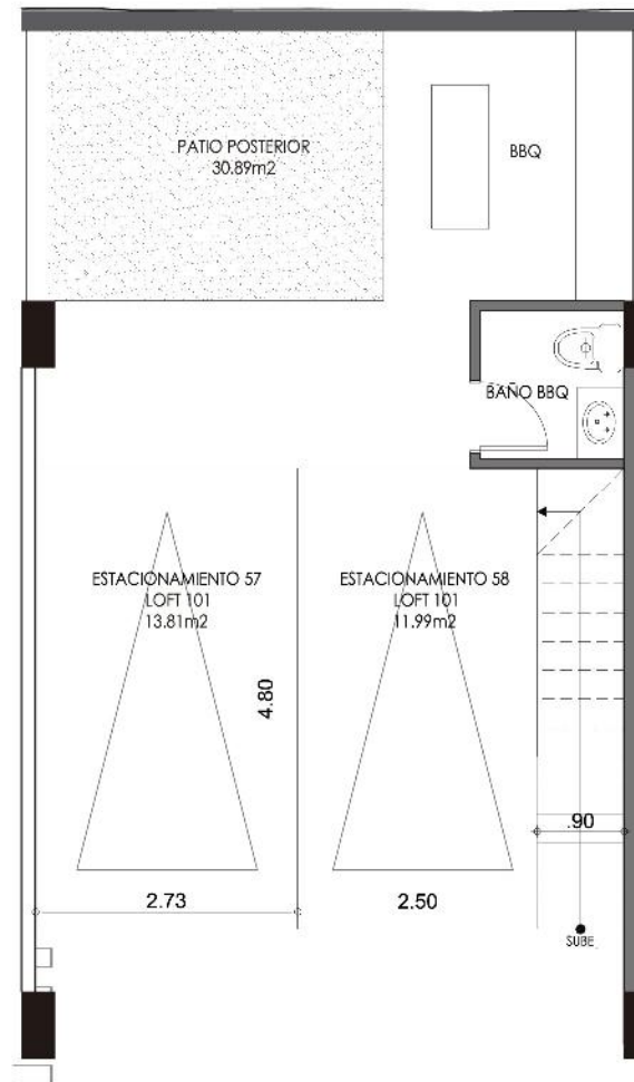
PLANTA BAJA
