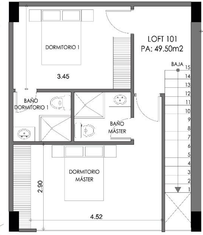
PLANTA ALTA
