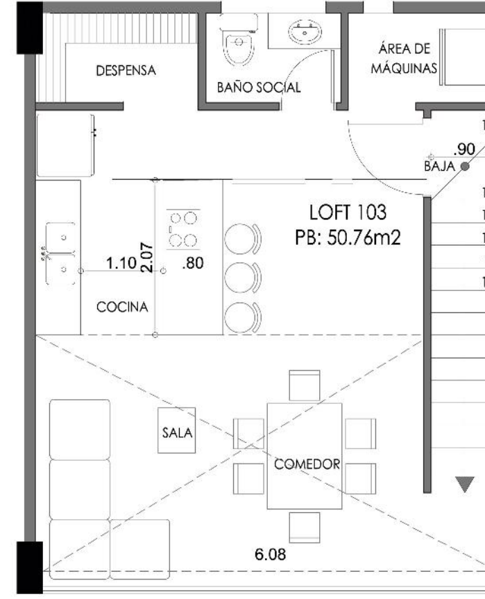
PLANTA BAJA
