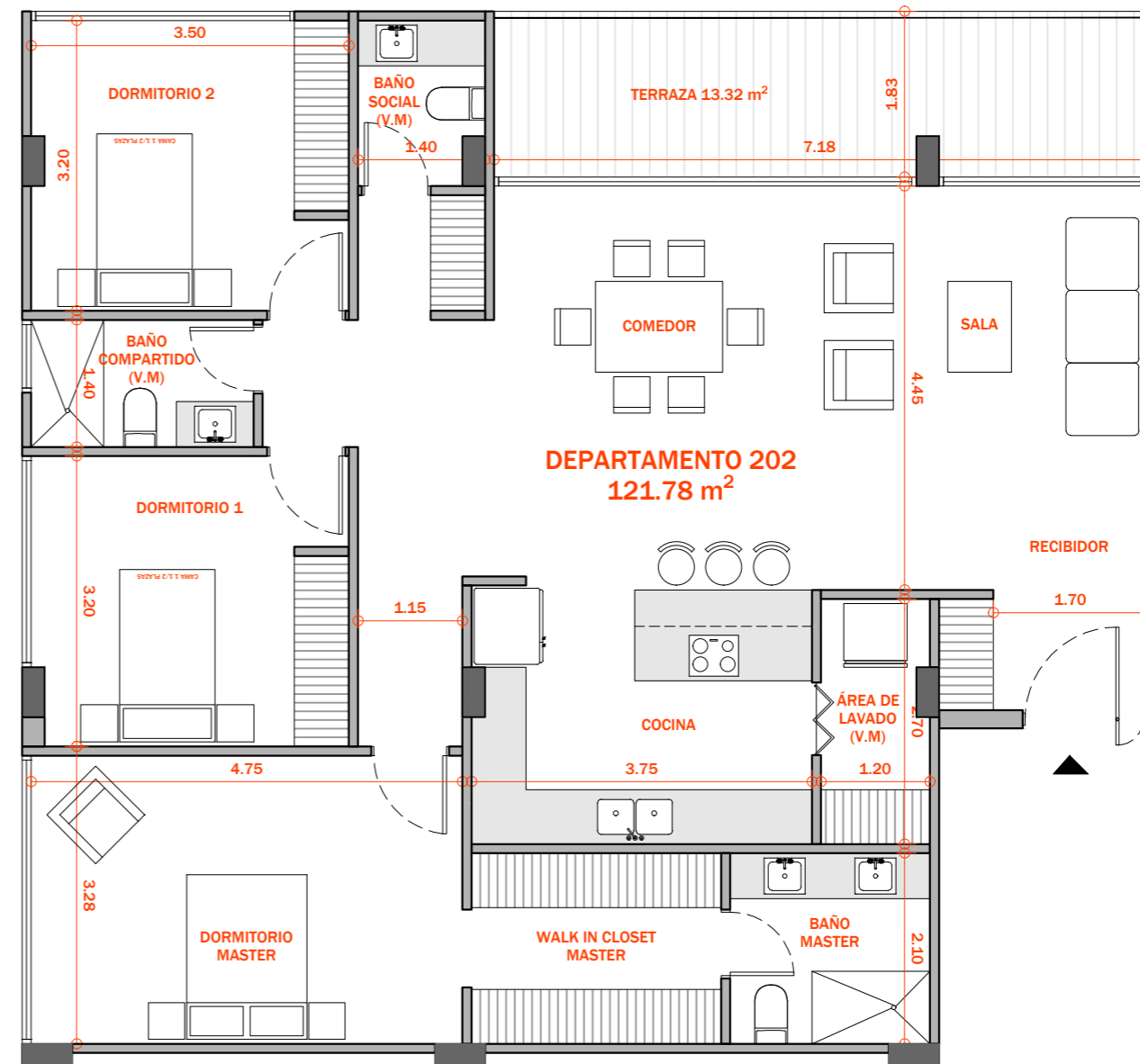
DEPARTAMENTO 202 - 302 ESC 1:75
