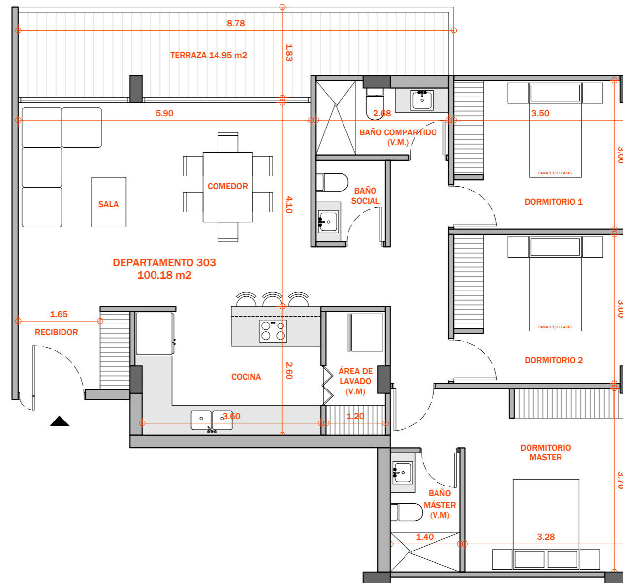
DEPARTAMENTO 303 ESC 1:75
